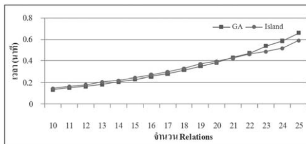
ภาพที่ 3 ผลการเปรียบเทียบประสิทธิภาพด้านเวลาในช่วง 10 ถึง 25 รีเลย์ชัน
