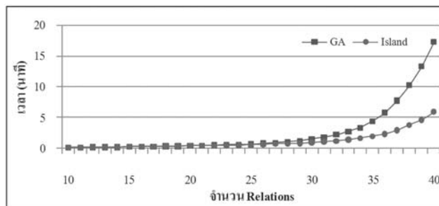
ภาพที่ 2 ผลการเปรียบเทียบประสิทธิภาพด้านเวลาระหว่าง Island based PGA และ GA
