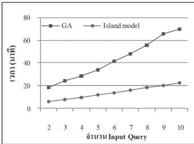
ภาพที่ 5 เปรียบเทียบประสิทธิภาพด้านการรองรับปริมาณงานจำนวนมากระหว่าง GA และ Island-based PGA
