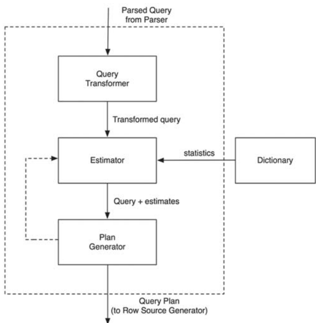
ภาพที่ 1 กระบวนการค้นหาคำถามที่เหมาะสมที่สุดแบบกระจาย
