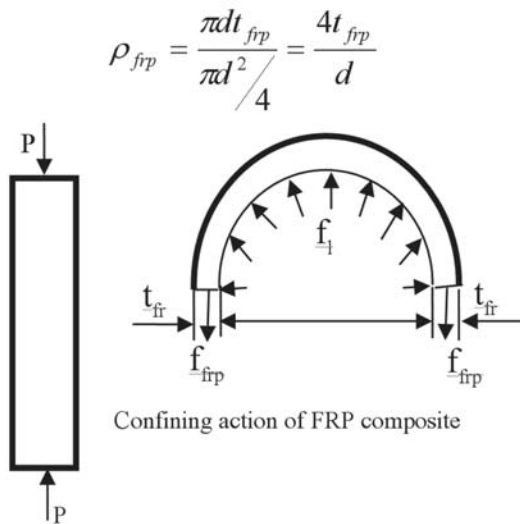
ภาพที่ 1 พฤติกรรมของคอนกรีตหน้าตัดกลมที่ถูกโอบรัดด้วยคาร์บอนไฟเบอร์ (J.G. Teng, J.F.Chen, S.T.Smith, L.Lam, 2002)
